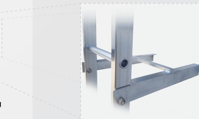
Obr.: Sklopná podpera
