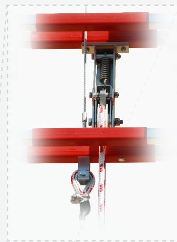
Obr.: Brzda lana
